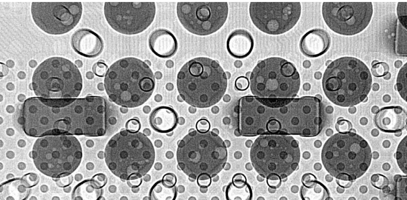
BGAとバンプの2D概要
